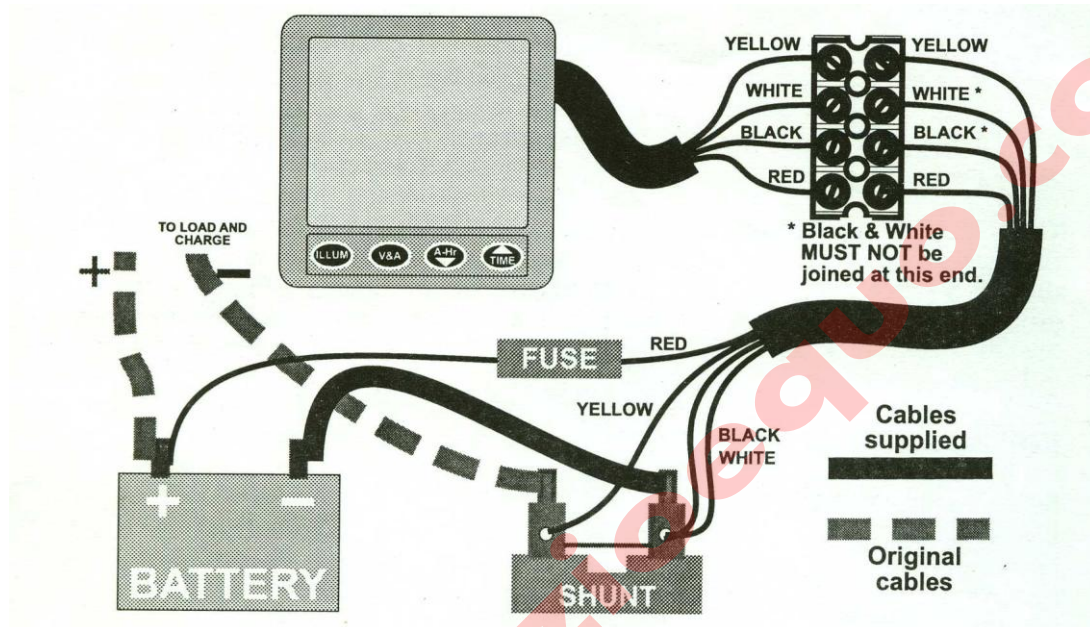
Figura 1 - Collegamento dei cavi
